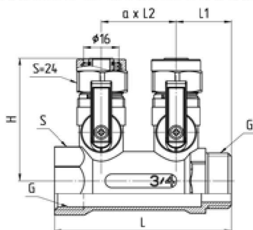
Рисунок 2 – Габаритные размеры коллектора
